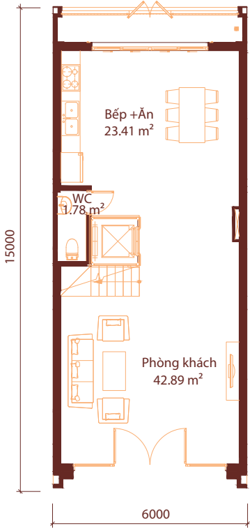
Mặt bằng tầng 1
