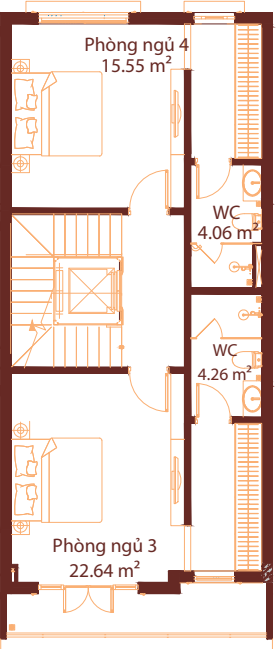
Mặt bằng tầng 3
