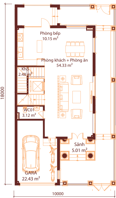
Mặt bằng tầng 1
