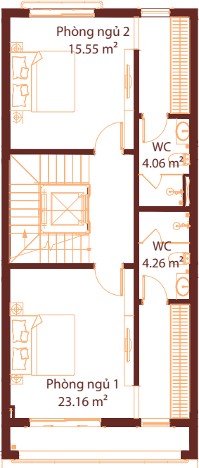
Mặt bằng tầng 2
