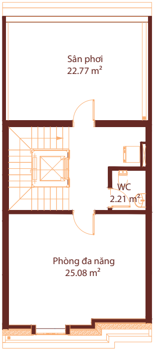
Mặt bằng tầng 4
